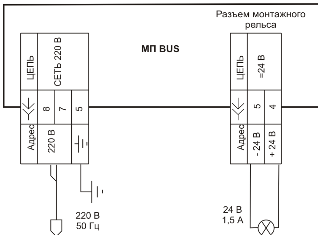
Рисунок 5.1 – Схема соединений МП BUS
